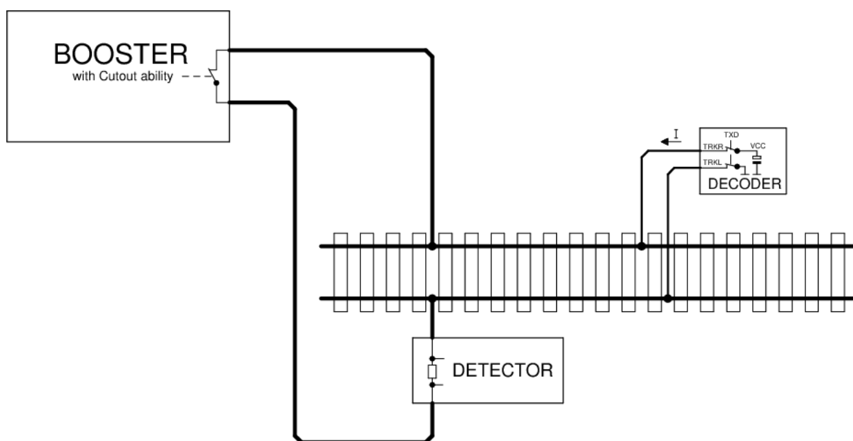
Bild 1: RailCom Prinzipschaltbild
