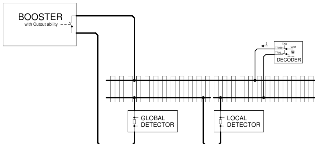
Bild 5: Lokalisierung Fahrzeugdecoder
