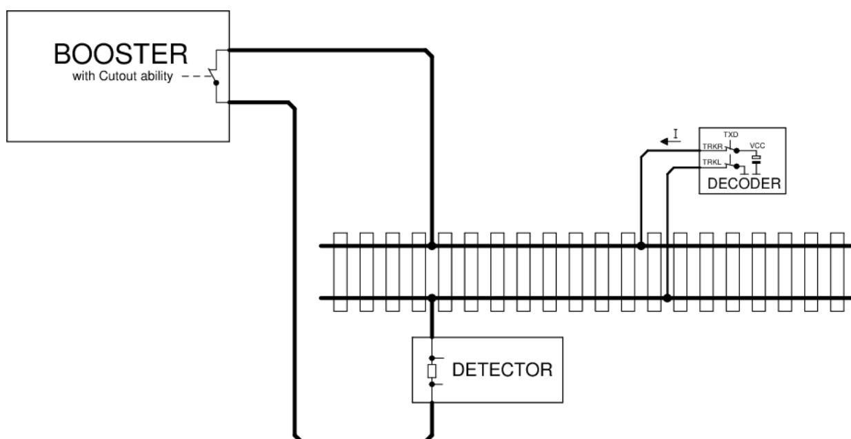
Bild 1: RailCom Prinzipschaltbild
