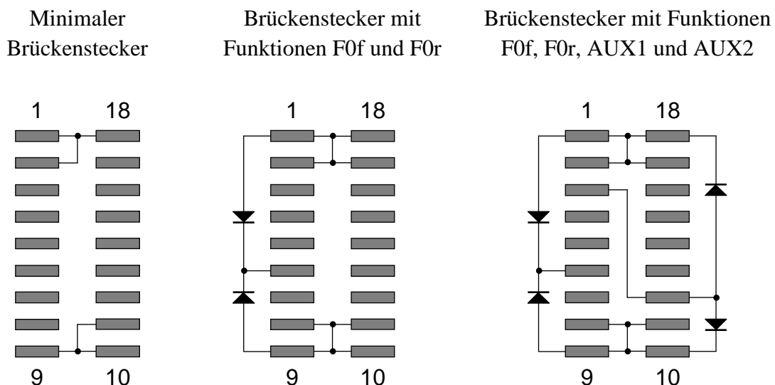
Bild 5: Typische Brückenstecker.
