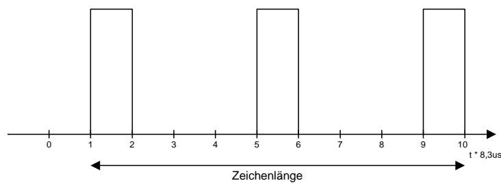
Synchronzeichen
