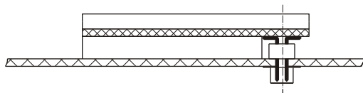
Bild 4: Einbau in kompakter Variante
